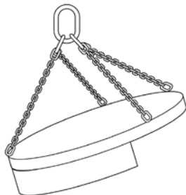
Figure 14: Toute la charge est supportée par 1 brin
